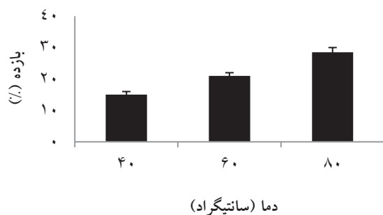
شکل ۳- تأثیر زمان و دمای استخراج بر بازده عصاره بدست آمده از گیاه دارویی چویل به روش رفلکس
